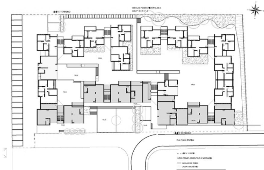
Figura 5 Planta baixa e implantação esquemáticas do projeto habitacional Jardim Nazareth, em Suzano-SP, de 2010, de 55 UHs de 2 e 3 quartos, com 59m 2 e 64m 2 , financiado pelo Programa Minha Casa Minha Vida do Governo Federal. Fonte: < http://www.usinactah.org.br/index.php?/arquivo/jd-nazareth/ >. Acesso em: 18 mai. 2012.
