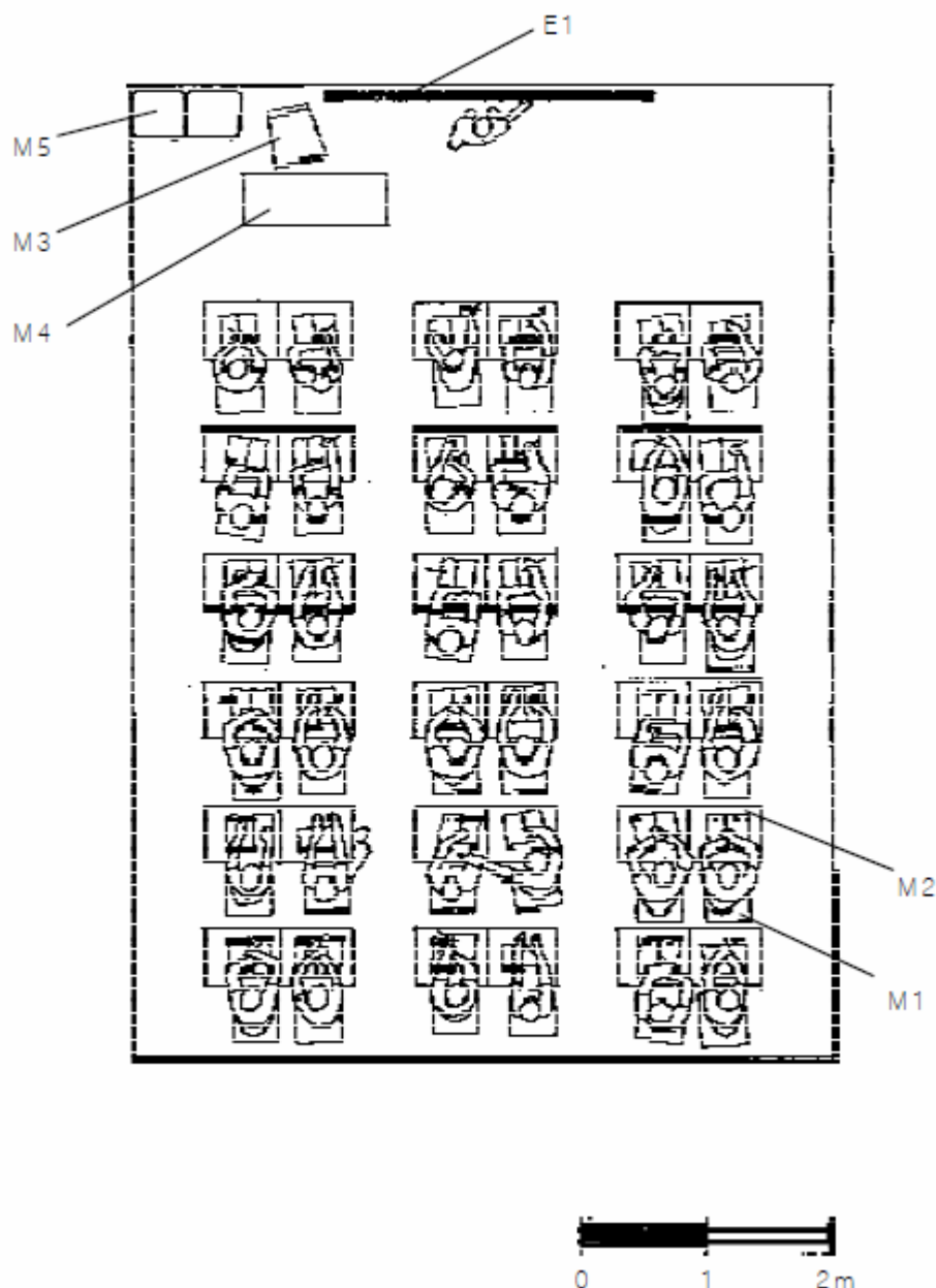
Figura 3 Diagrama de sala de aula para ensino fundamental, com 46,98 m 2 , equipada com quadro de giz (E1), cadeira para aluno (M1), mesa para aluno (M2), cadeira do professor (M3), mesa para professor (M4) e armário de aço (M5). Fonte: MEC. Espaços educativos para ensino fundamental. Subsídios para elaboração de projetos e adequação de edificações escolares. 124 f. Brasília: FUNDESCOLA; MEC, 2002. (Série cadernos técnicos, n. 4). v. 2.
